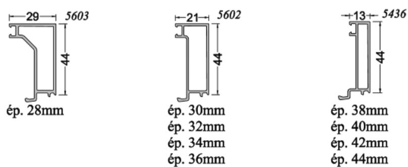
PARECLOSE FIXE
