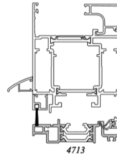
PORTE D'ENTRÉE
