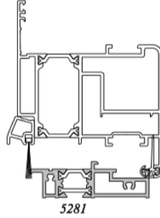
PORTE FENETRE à barillet
