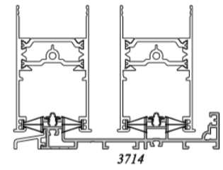
COULISSANT (uniquement 2 vantaux)
