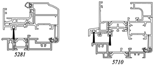
FRAPPE Ouvrant Caché Ouvrant Visible
