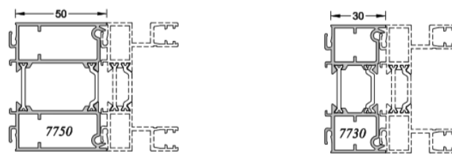
ÉLARGISSEUR
