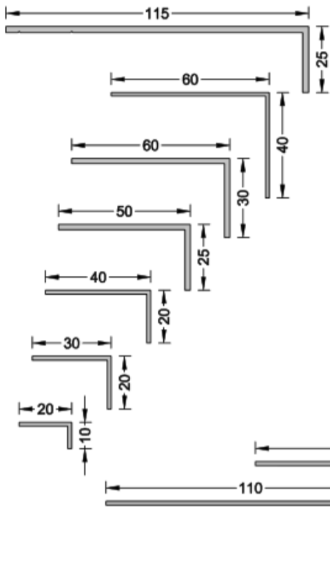
CORNIERES
