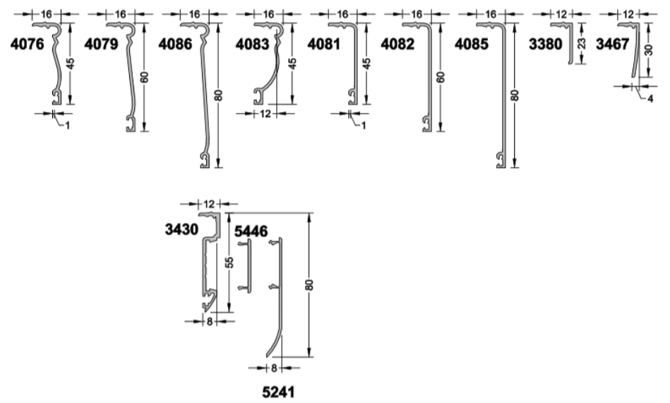
COUVRE-JOINTS
