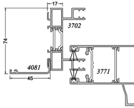
Couissant SÉPALUMIC 70
