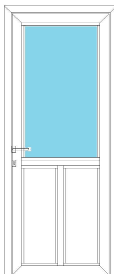
1 vitrage + 1 traverse + 1 meneau + 2 panneaux (lisse ou plate-bande)
