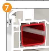
Renfort acier suivant abaques SCHÜCO
