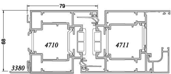
Porte d'Entrée SÉPALUMIC 70
