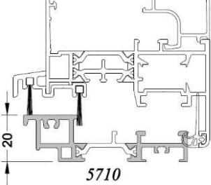
Ouvrant Visible
