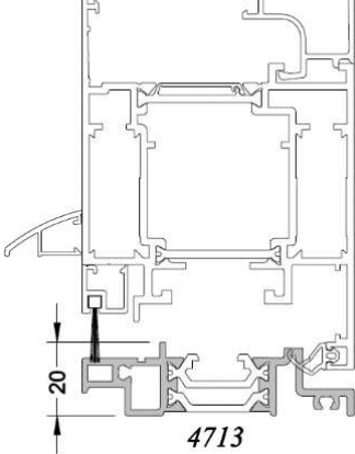
PORTE D'ENTRÉE
