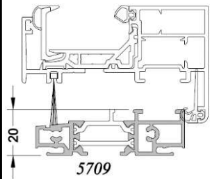
FRAPPE Ouvrant Caché
