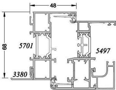
SÉPALUMIC 70 Ouvrant Visible
