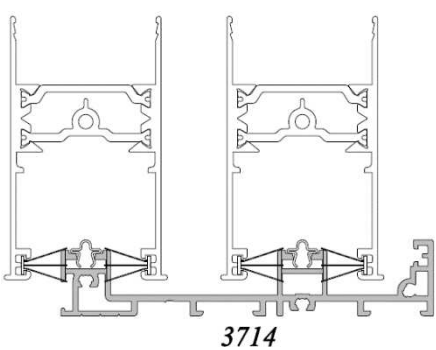
COULISSANT (uniquement 2 vantaux)
