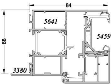
SÉPALUMIC 70 Ouvrant Caché
