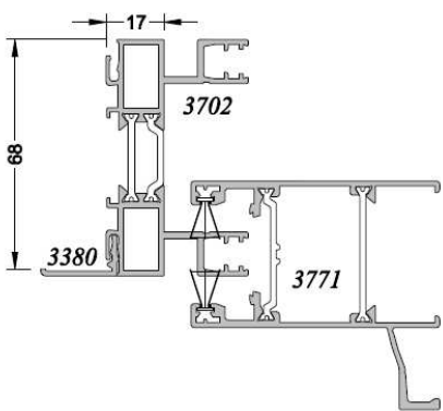
Coulissant SÉPALUMIC 70
