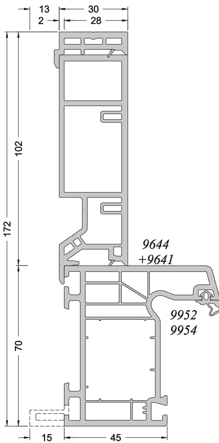
DU68 ou DN68 + T102
