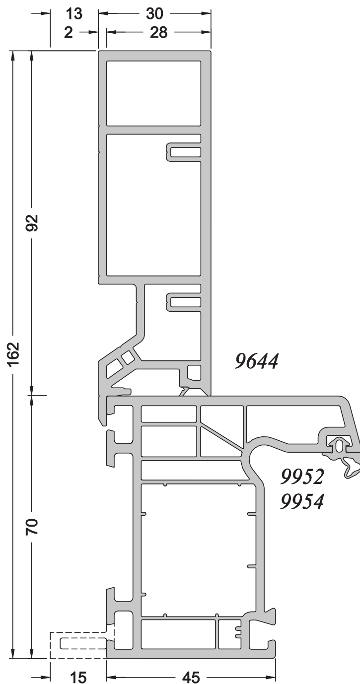
DU68 ou DN68 + T92
