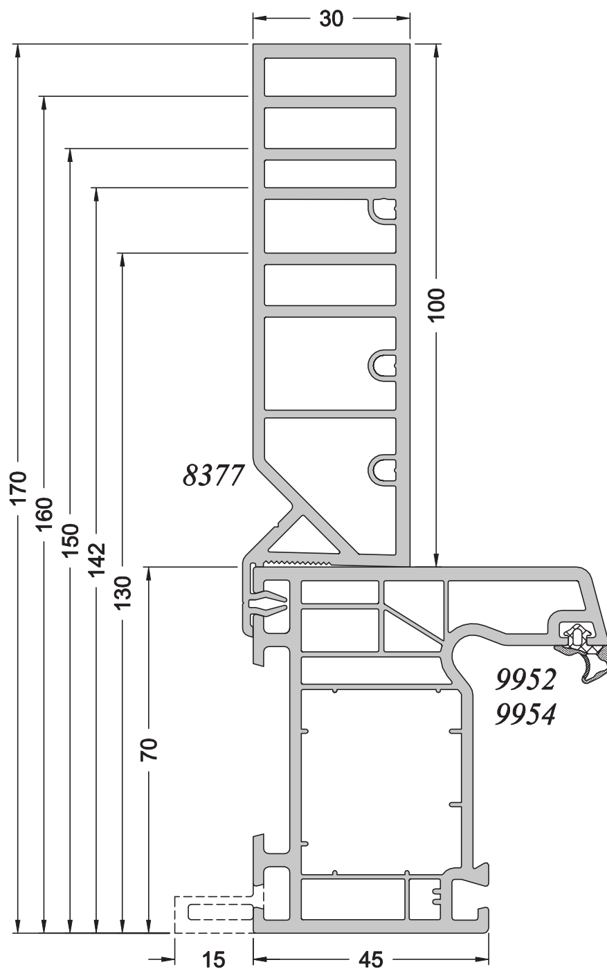
DU68 ou DN68 + T100
