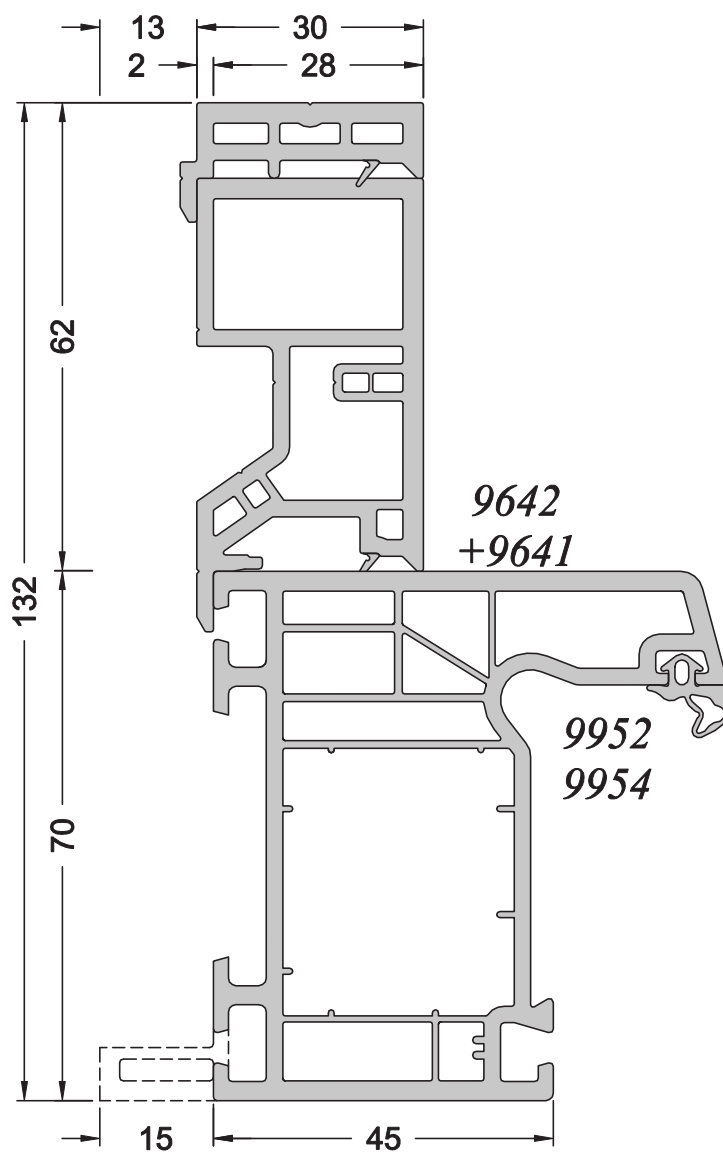
DU68 ou DN68 + T62
