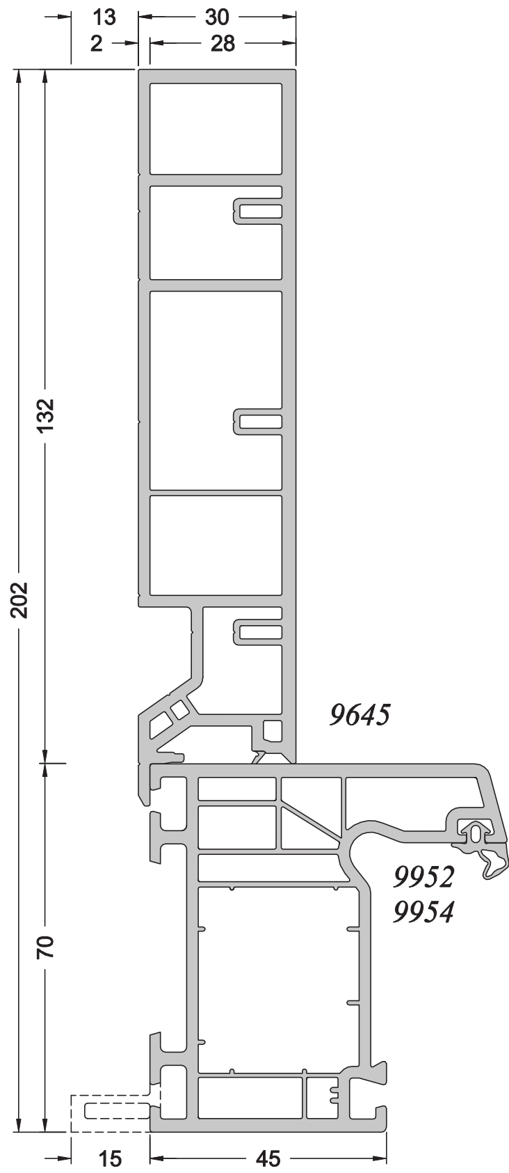
DU68 ou DN68 + T132
