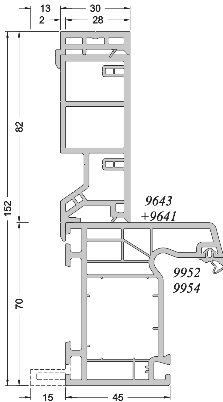
DU68 ou DN68 + T82
