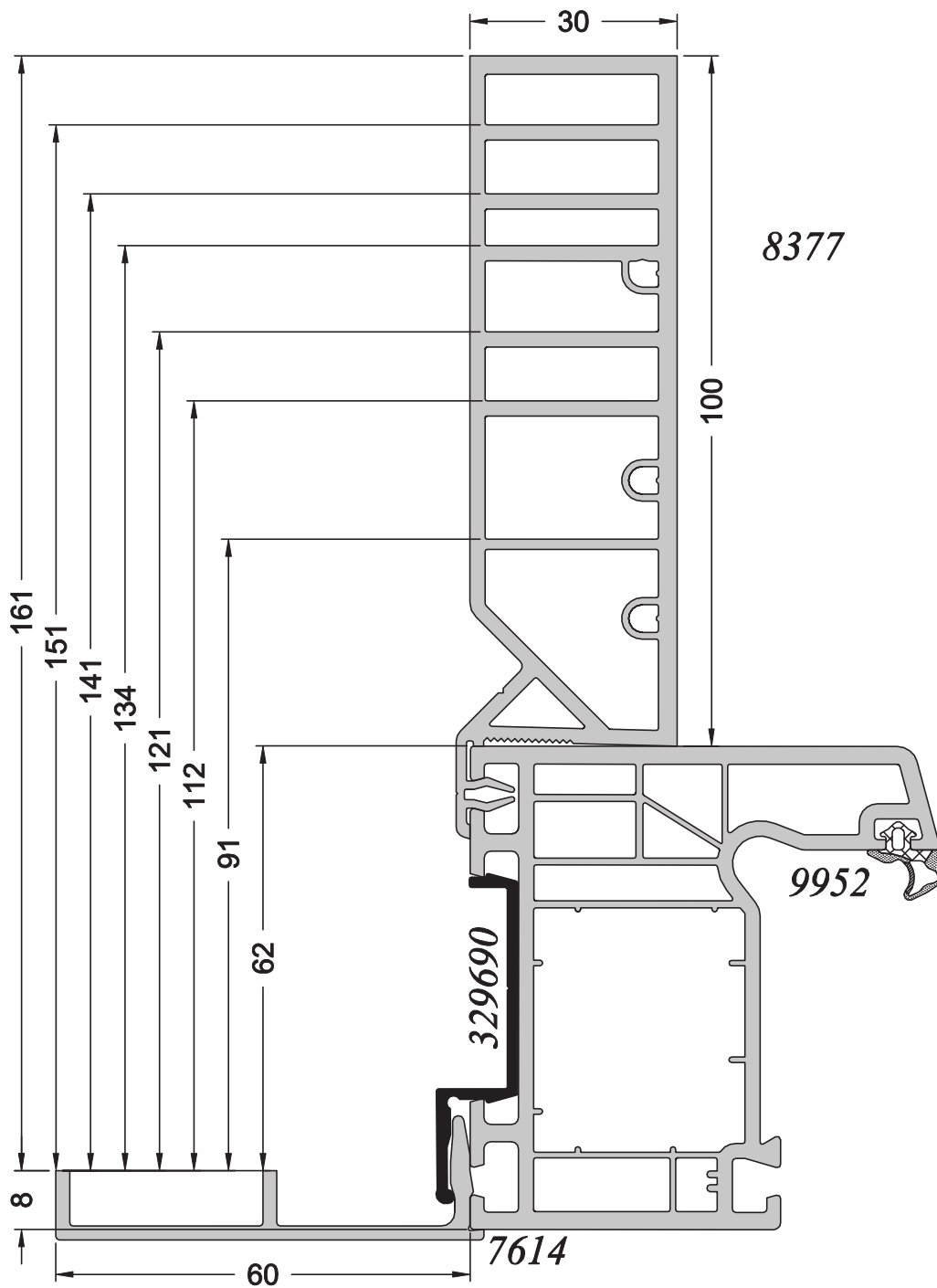
DU68 + Profilé d'adaptation + Couvre-Joint rapporté 60 + T100
