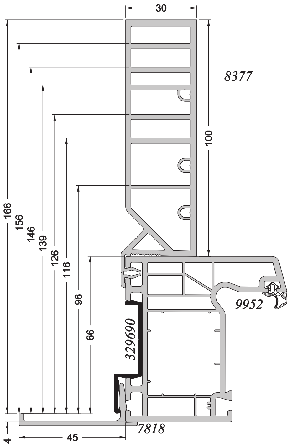
DU68 + Profilé d'adaptation + Couvre-Joint rapporté 48 + T100
