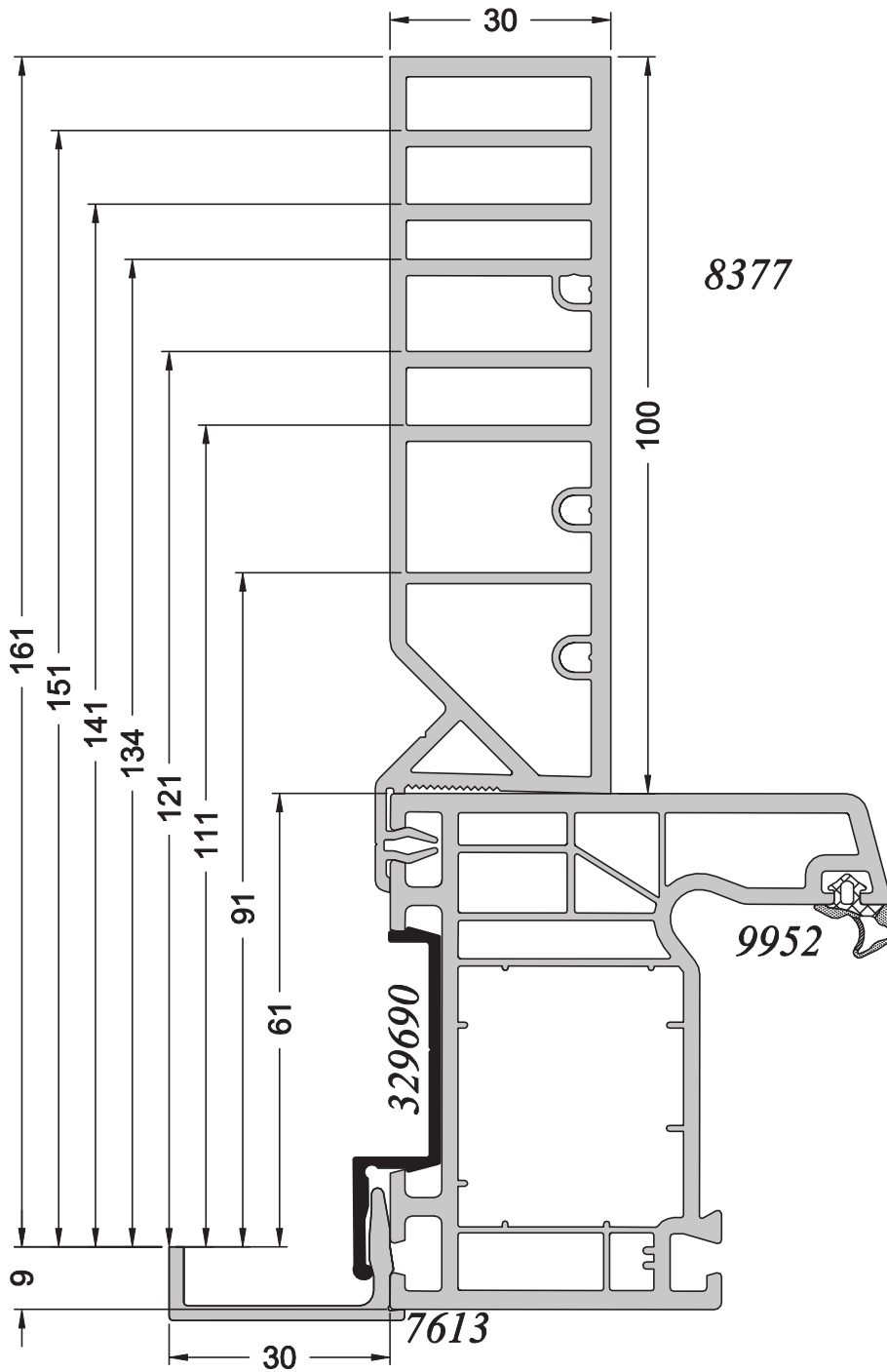
DU68 + Profilé d'adaptation + Couvre-Joint rapporté 30 + T100
