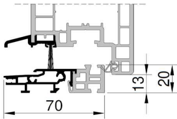
Seuil 20mm
