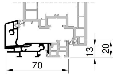
Seuil 40mm
