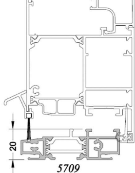
PORTE FENÊTRE à barillet
