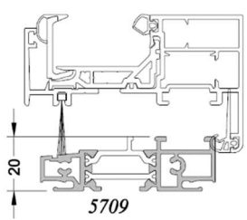
FRAPPE Ouvrant Caché
