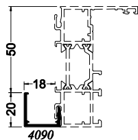
Compensateur
